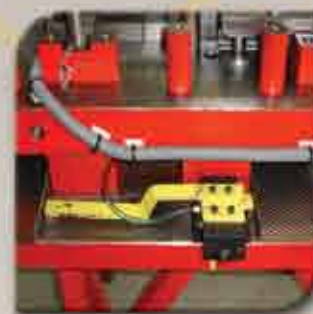
Vibrating systems for scrap release Sistemas de vibración para salida de chatarra
